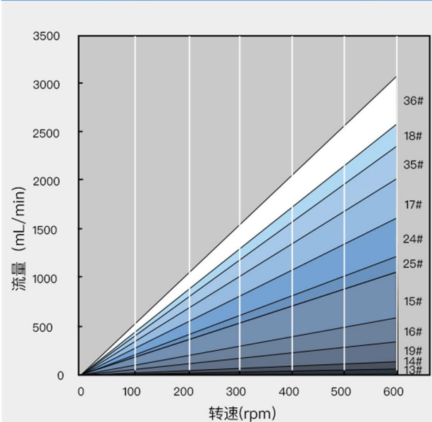
EasyPump泵头流量范围（0.1-600rpm）
