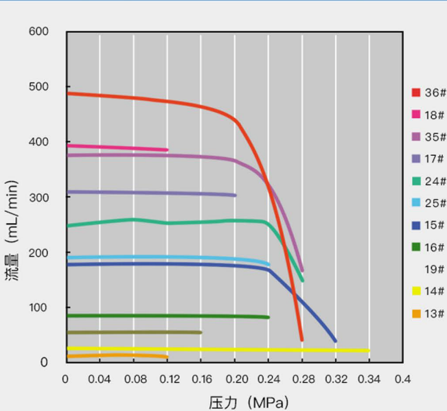
EasyPump泵头压力/流量曲线图(100rpm)
